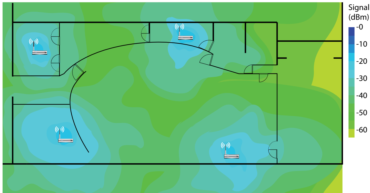
Abbildung.: Graphische Darstellung einer Funkausleuchtung
